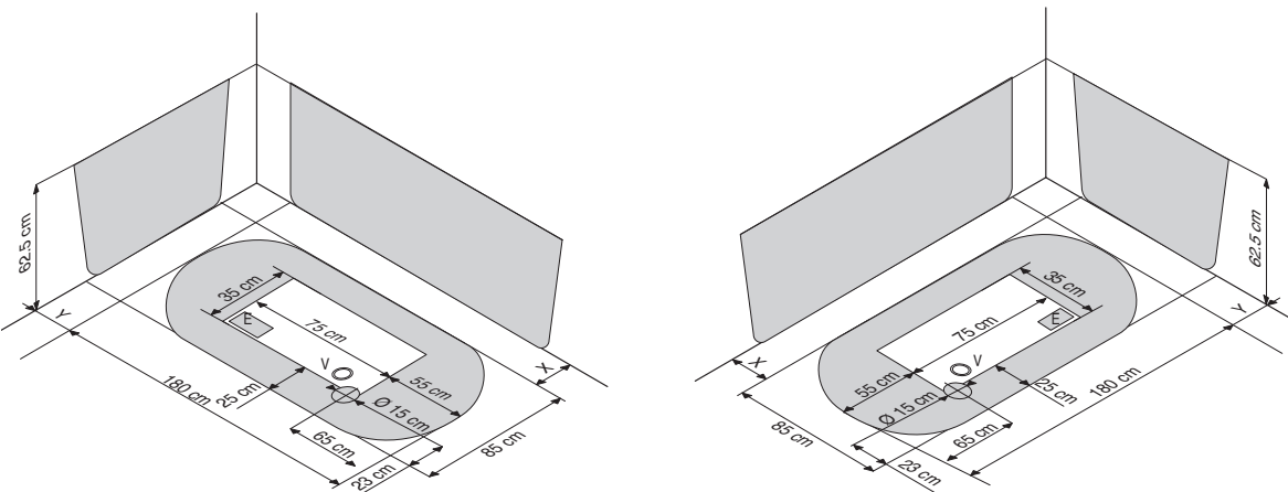
Schéma technique de pré-installation (en cm)
