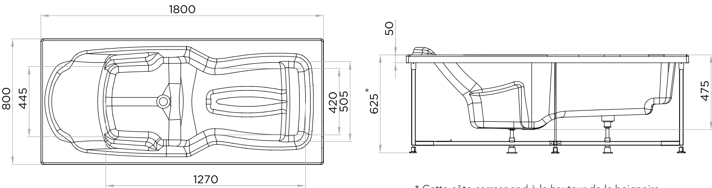
Dimensions de la baignoire (en mm)
