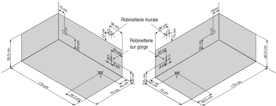
Emplacement des injecteurs et buses, selon le système
